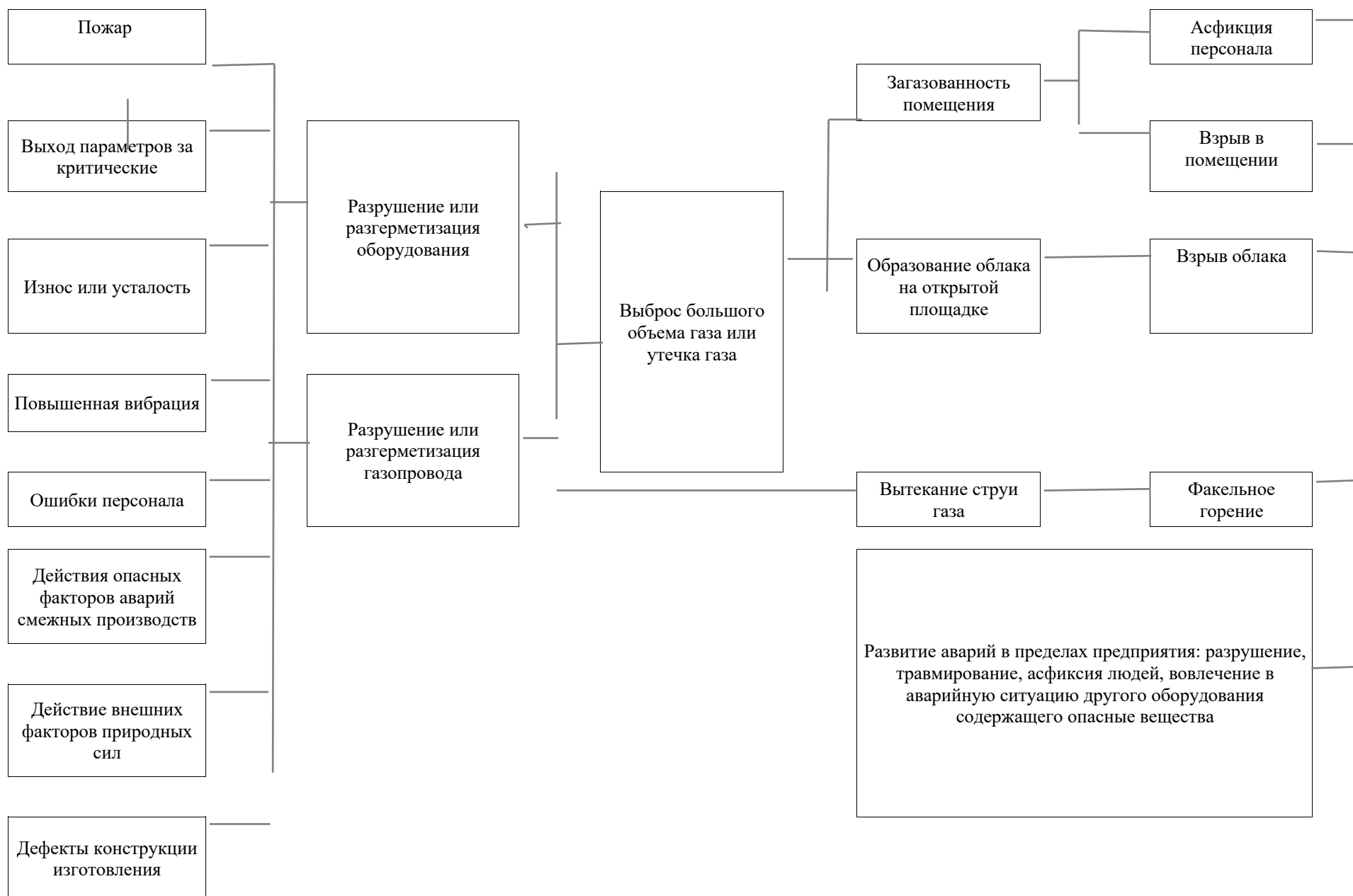
Рисунок 1. Блок-схема сценариев возникновения аварийных ситуаций на котельной пос. Лесосплава, д.28, г. Кольчугино
